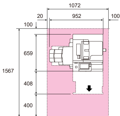
● Model-F/PF +サイドトレイ
