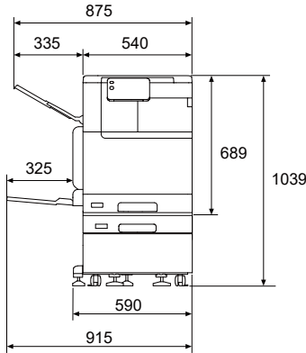
● Model-DC +キャビネット付き1トレイモジュール +サイドトレイ
