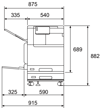
● Model-DC +1トレイモジュール +キャスター +サイドトレイ
