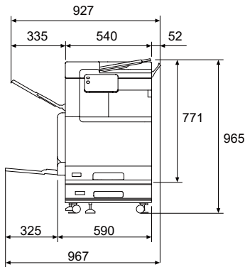
● Model-F/PF +1トレイモジュール +キャスター +サイドトレイ
