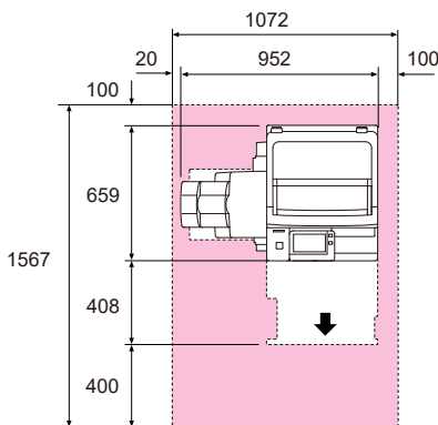
● Model-DC +サイドトレイ
