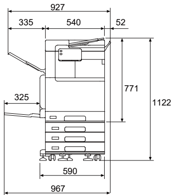
● Model-F/PF +3トレイモジュール +サイドトレイ
