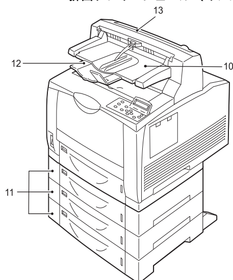
標準モデル + トレイモジュール (オプション) 3 段 + 排出トレイモジュール (オプション)
