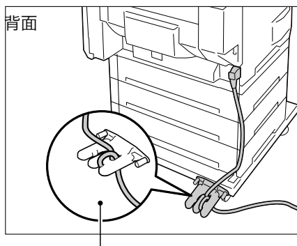
電源コードをケーブルフックに巻き付けた状態
