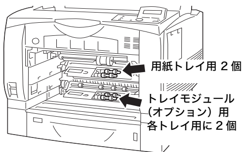
プリンター内部
