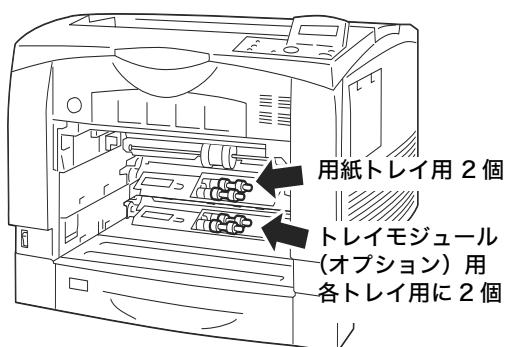
プリンター内部
