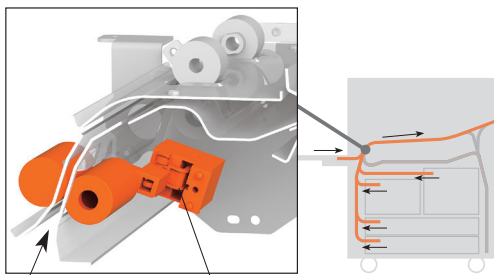
用紙搬送 重送検知センサー ローラー間隔の変動を監視します。
